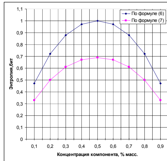
Рис. 1 - Зависимость энтропии от концентрации
