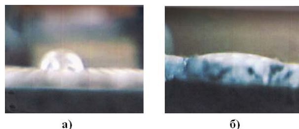
Рис. 3 - Растекание капли по СВМПЭ поверхности до (а) и после (б) обработки в ВЧЕ-разряде при J_a=0,7 А, U_a=5 кВ ( \tau=180 с; P=26,6 Па; G_{аргон} = 0,04 г/с)
