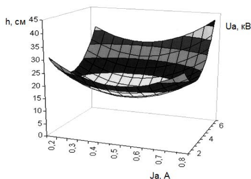
Рис. 1 - Поверхность отклика на плоскости при постоянном значении \tau=180 с (ткань из волокна SK 75)
