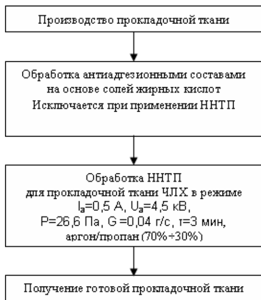
Рис. 1 – Вариант технологической схемы активации прокладочных тканей с применением ННТП
