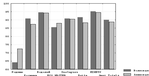
Рис. 1 – Эффективность различных фильтров по очистке воды от ионов Sr, %
