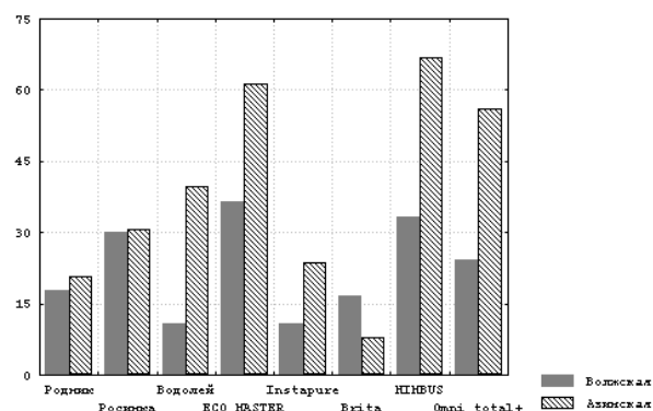
Рис. 3 – Сравнение эффективности различных типов фильтров по снижению жесткости воды, %
