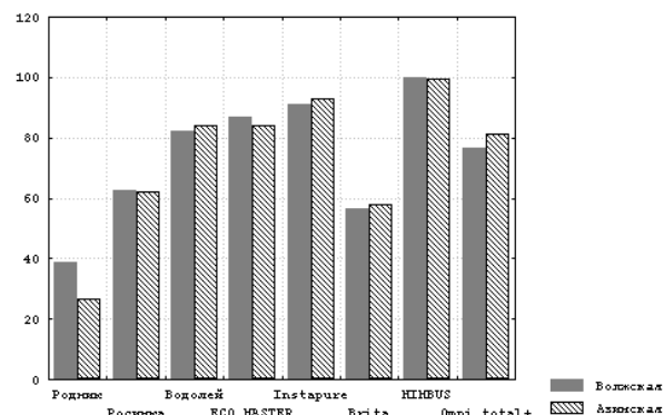
Рис. 2 – Сравнение эффективности различных типов фильтров по очистке воды от ионов Fe, %
