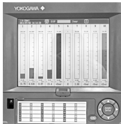
Рис. 2 - Станция сбора данных CX2020
