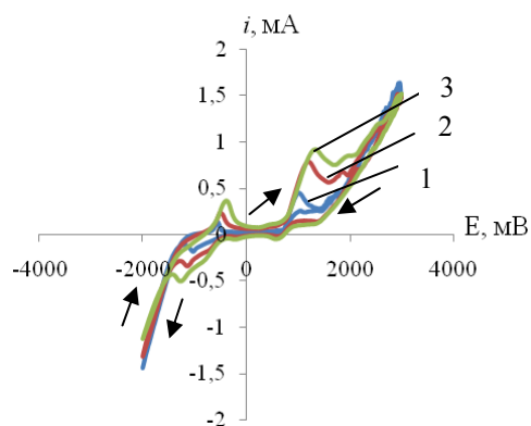
Рис. 3 - Циклическая вольтамперограмма стального электрода (X18H10T) в 0.01 M растворе NaOH (1 – 10 мВ/с, 2 – 50 мВ/с, 3 – 100 мВ/с)
