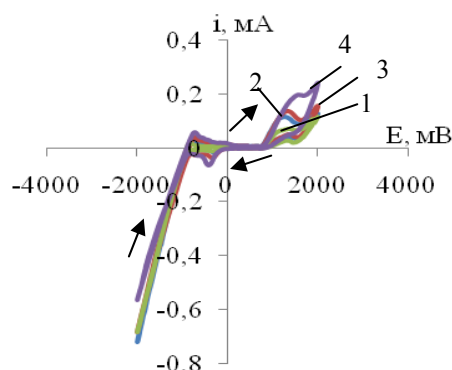
Рис. 4 - Циклическая вольтамперограмма платинового электрода в водном растворе 0.01M NaOH + натриевая соль 3,4-дигидрокси-9,10-диоксоантраценсульфоновая-2 кислота (0.01 г/л) при скорости развертки потенциала, мВ/с: 1 – 10; 2 – 25; 3 – 50; 4 – 100
