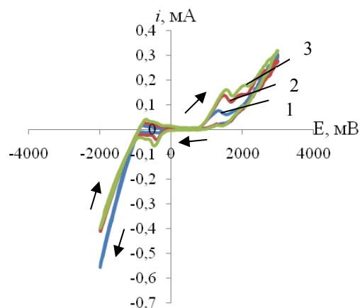
Рис. 2- Циклическая вольтамперограмма платинового электрода в 0.01 М растворе \text{NaOH} (1 – 10 мВ/с, 2 – 50 мВ/с, 3 – 100 мВ/с)
