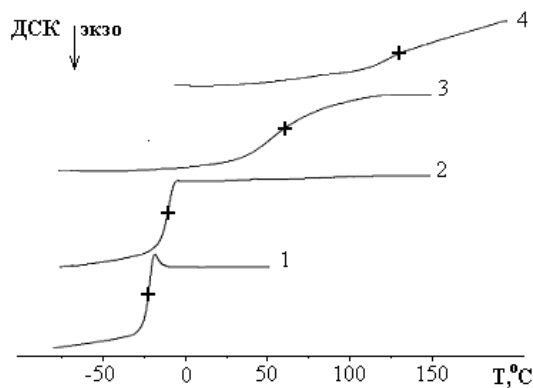
Рис. 4 - Термограммы ДСК аддуктов. Степени конверсии: 0% (1), 20% (2), 60% (3) и 100% (4)
