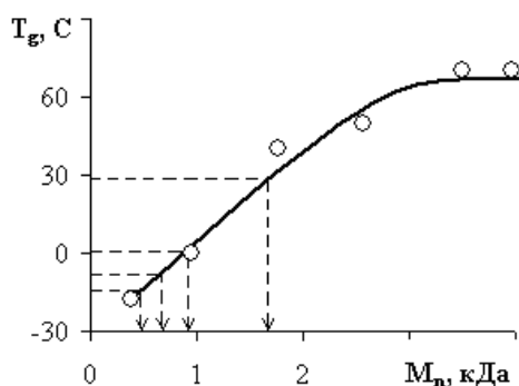
Рис. 1 - Молекулярная зависимость температур стеклования эпоксидных олигомеров [Шмалий, Жаворонок]. Пояснение в тексте
