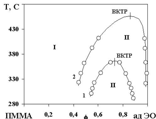
Рис. 5 - Диаграммы фазовых состояний систем ПММА (15000)–адЭО: \alpha : 1 – 0,3; 2 – 0,4 . Области растворов I и гетерогенного состояния - II
