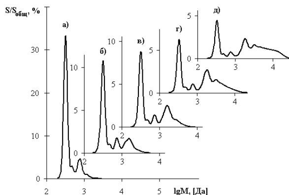
Рис. 2 - Молекулярно массовые распределения аддуктов ЭО, приготовленных при использовании ДДС. Предполагаемые степени конверсии: а) 0%, б) 5%, в) 10%, г) 20%, д) 30%
