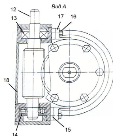
Рис. 3 - Конструкция экструзионной головки для изготовления извитых изделий из термопластов
