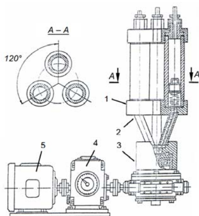
Рис. 1 - Установка для изучения слойно-секторного извитого течения комбинированных расплавов полимеров (по А. С. СССР №994283): 1 - цилиндр высокого давления; 2 - соединительный блок; 3 - экструзионная головка; 4 - вариатор; 5 - электродвигатель
