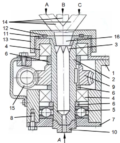
Рис. 2 - Конструкция экструзионной головки для изготовления извитых комбинированных изделий из различных термопластов: 1 - разъемный корпус; 2 - вращающийся цилиндр; 3 - треугольные выступы; 4 - радиальный подшипник; 5 - упорный подшипник; 6 - втулка; 7 - крышка; 8 - болт; 9 - червячное колесо; 10 - формующий канал; 11 - переходной диск; 12 - уплотнительное кольцо; 13 - крышка; 14 - подводящие патрубки; 15 - червяк; 16 - коническая камера. А, В, С - расплавы полимеров
