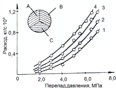
Рис. 5 - Зависимости расхода комбинированных полимеров от перепада давления при разных частотах вращения канала: А – ПВД марки 10802-020; В – ПВД марки 15802-020; С – ПВД марки 176-901; частота вращения: 1 - n=0 об/с; 2 - n=10 об/с; 3 - n=22 об/с; 4 - n=30 мин -1
