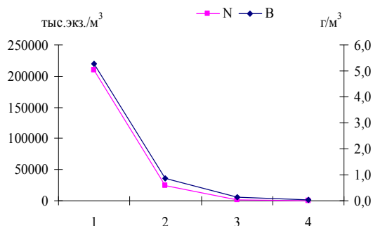
Рис. 1 - Динамика численности и биомассы инфузорий, в контроле ПВ: 1 – май, 2 – июнь, 3 – июль, 4 – сентябрь
