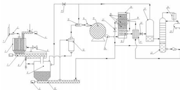
Рис. 3 - Схема установки по получению метанола из древесных отходов
