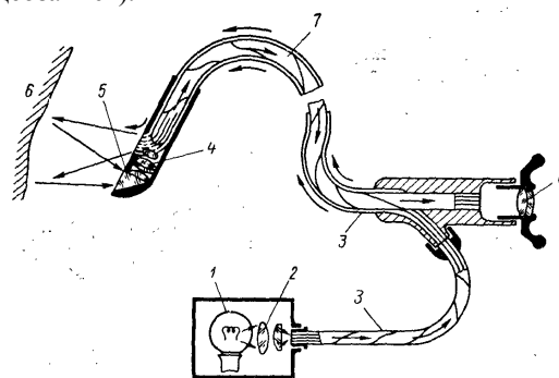
Рис. 1 - Схема устройства гибкого эндоскопа с волоконным световодом: 1- лампа осветителя; 2- конденсор; 3 - осветительный жгут; 4 объектив; 5 - призма; 6 – объект наблюдения; 7 – жгут, передающий изображение; 8 - окуляр
