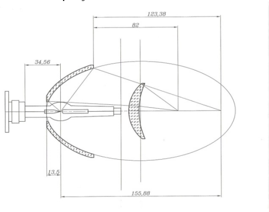
Рис. 2 - Оптическая схема осветителя ксенонового ОКЭ-250
