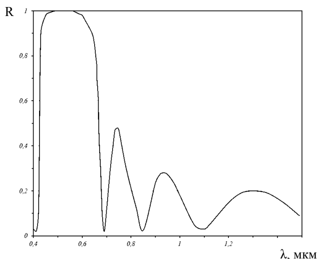
Рис. 3 - Спектральная зависимость коэффициента отражения «холодного» зеркала
