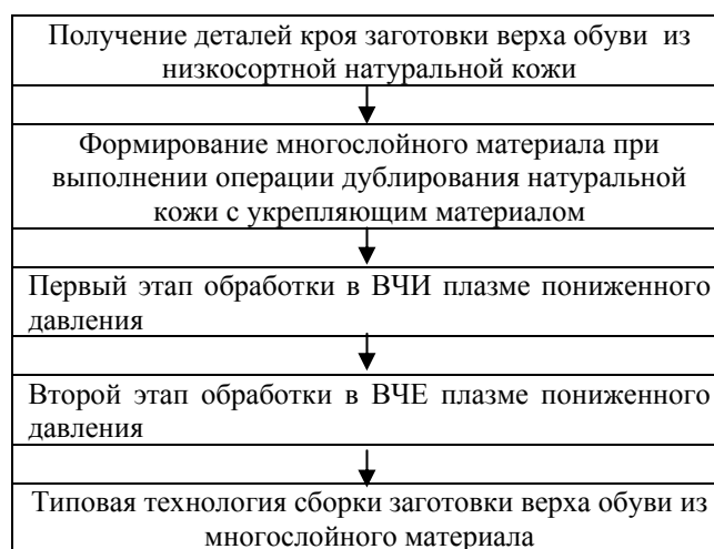
Рис. 1 – Технологический процесс производства заготовки верха обуви из комплексного материала из низкосортной натуральной кожи с последовательным применением ВЧ плазмы индукционного и емкостного разрядов пониженного давления
