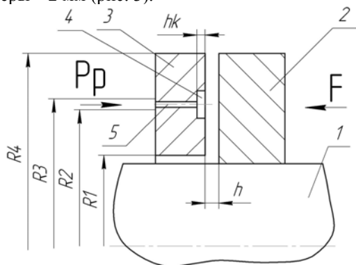
Рис. 2 - Схема подшипника: 1 – ротор; 2 - упорный диск; 3 - рабочая поверхность подшипника; 4 - камера нагнетания; 5 - дроссель
