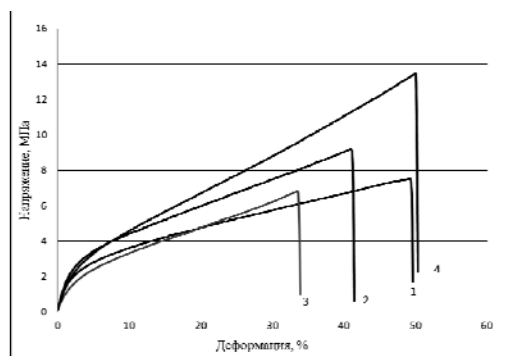
Рис. 3 - Диаграмма напряжение-деформация биопленок на основе картофельного крахмала, обработанного пуллулазой
