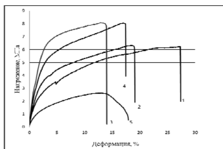
Рис. 1 - Диаграмма напряжение-деформация биопленок на основе картофельного крахмала, обработанного при 90°C
