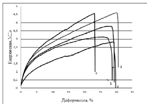
Рис. 2 - Диаграмма напряжение-деформация биопленок на основе картофельного крахмала, обработанного при 120°C
