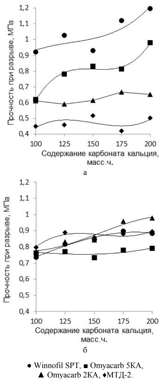
Рис. 1 – Влияние содержания и дисперсности наполнителей на когезионную прочность неотверждаемых композиций с БНК-18 (а) и БНК-40 (б)
