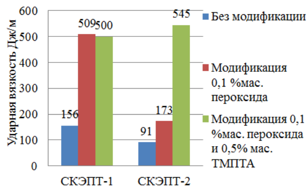
Рис. 2 - Диаграмма зависимости ударной модификации от способа модификации бинарных смесей ПП/СКЭПТ состава 80/20 для двух типов каучуков
