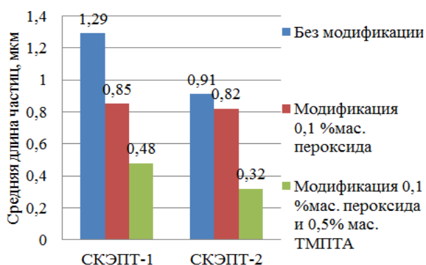
Рис. 1 - Диаграмма зависимости средней длины частиц от способа модификации бинарных смесей ПП/СКЭПТ состава 80/20 для двух типов каучуков
