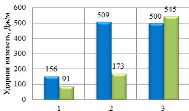
Рис. 2 - Зависимость ударной вязкости композиций ПП/СКЭПТ от состава модифицирующих агентов: 1 – немодифицированная система, 2- модификация пероксидом 0,1 % мас., 3- модификация системой пероксид 0,1 %мас./ТМПТА 0,5 % мас. ■ - СКЭПТ-1, ■ - СКЭПТ-2
