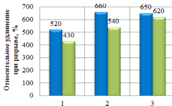
Рис. 4 - Зависимость удлинения при разрыве композиций ПП/СКЭПТ от состава модифицирующих агентов: 1 – немодифицированная система, 2- модификация пероксидом 0,1 % мас., 3- модификация системой пероксид 0,1 %мас./ТМПТА 0,5 % мас. ■ - СКЭПТ-1, ■ - СКЭПТ-2
