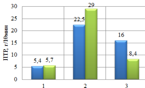
Рис. 1 - Зависимость ПТР композиций ПП/СКЭПТ от состава модифицирующих агентов: 1 – немодифицированная система, 2- модификация пероксидом 0,1 % мас., 3- модификация системой пероксид 0,1 %мас./ТМПТА 0,5 %мас. ■ - СКЭПТ-1, ■ - СКЭПТ-2
