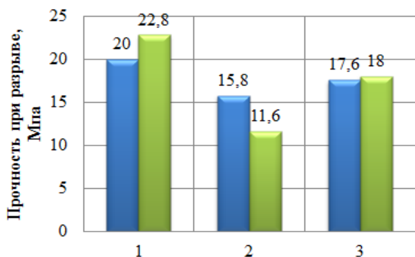
Рис. 3 - Зависимость прочности при разрыве композиций ПП/СКЭПТ от состава модифицирующих агентов: 1 – немодифицированная система, 2- модификация пероксидом 0,1 %мас., 3- модификация системой пероксид 0,1 %мас./ТМПТА 0,5 % мас. ■ - СКЭПТ-1, ■ - СКЭПТ-2
