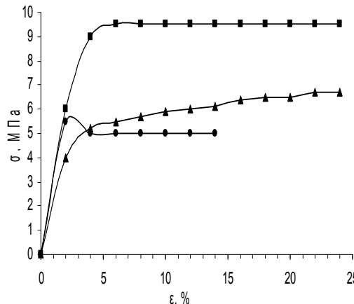
Рис. 4 - Кривые напряжение-деформация для образцов ДАЦ
