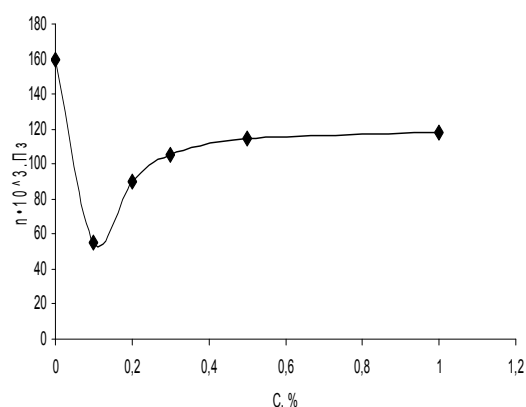
Рис. 1 - Кривая зависимости вязкости расплава ДАЦ от содержания АМПИК (температура расплава 190 °С, нагрузка 10 кг)
