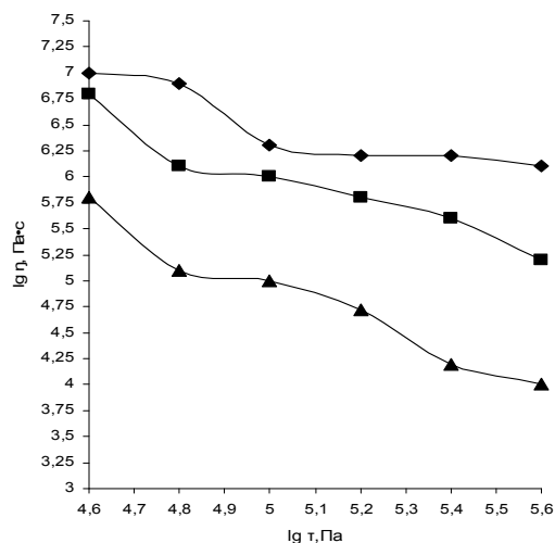
Рис. 2 - Кривые течения для расплава ДАЦ с ГМ-120 и АМПИКа (температура расплава 190 °С)
