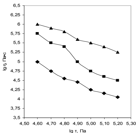
Рис. 3 - Кривые течения расплава этилцеллюлозы с кукурузным крахмалом (температура расплава 190 °С)
