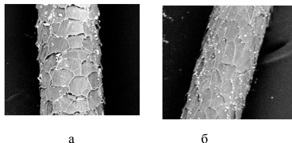
Рис. 4 – Микрофотографии поверхности волоса шубной овчины (×1500): а) без обработки; б) обработанный плазмой ВЧЕ разряда пониженного давления ( G_{Ar}=0,04 г/с, P=26,6 Па, Wp=0,9 кВт, t=3 мин)
