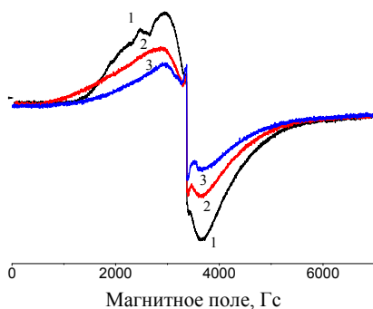
Рис. 4 - Спектры ЭПР исходного композита (1), после пропускания переменного тока с возрастающим напряжением от 0 до 220 В со ступенькой в 10 В и продолжительностью ступенек 1 мин в первый раз (2), во второй раз (3)
