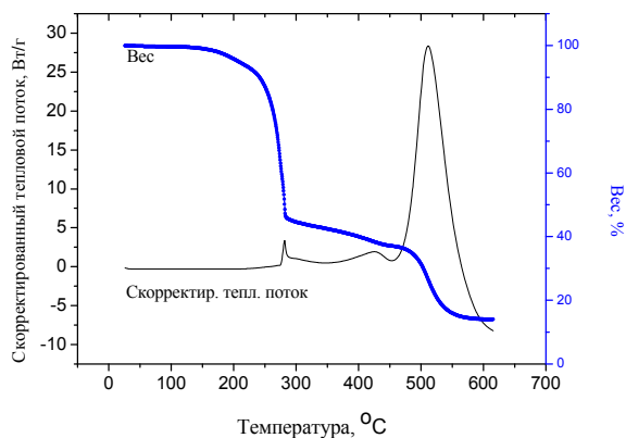
Рис. 5 - Результаты исследования композита совмещенным методом ДСК-ТГА
