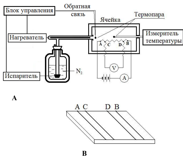
Рис. 1 - Схемы установки (А) и образца (В) композита для измерения температурной зависимости электрических характеристик проводящих эластомерных композитов потенциометрическим методом
