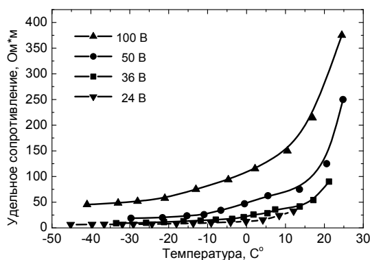
Рис. 2 - Графики зависимости удельного сопротивления композита от температуры при различных напряжениях
