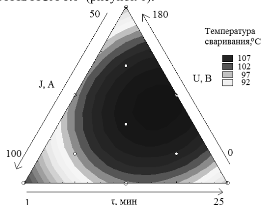
Рис. 1 – Оптимизация параметров нанесения плазменных конденсатов
