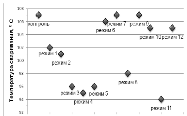
Рис. 2 – Изменение показателя температуры сваривания в зависимости от выбранного режима нанесения покрытия
