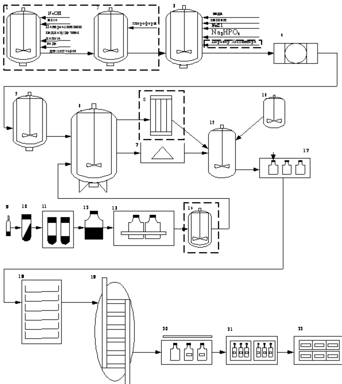
Рис. 1 - Аппаратурно-технологическая схема промышленного производства сухой живой вакцины против листериоза, сальмонеллеза или симбиотического препарата: 1 - реактор-гидролизатор; 2 - реактор для хранения осветленного гидролизата; 3 - реактор для приготовления питательной среды; 4 - мембранный фильтр; 5 - реактор для стерилизации питательной среды; 6 - биореактор (ферментер) для культивирования; 7 - ультрацентрифуга; 8 - установка для ультрафильтрации; 9 - ампула с лиофильно высушенным штаммом; 10 - штамм выращенный на скошенном агаре; 11 - штамм выращенный в жидкой питательной среде; 12 - штамм засеянный во флаконы 450мл; 13 - выращивание штамма во флаконах 450 мл на шуттель-аппарате в термостатируемом помещении; 14 - лабораторный ферментер для инокулята; 15 - емкость для смешивания биомассы с защитной средой высушивания; 16 - емкость для приготовления защитной среды высушивания; 17 - установка для фасовки и предварительной укупорки флаконов; 18 - низкотемпературный холодильник; 19 - сублимационная установка; 20 - полуавтоматическая линия укупорки, закатки флаконов, этикетирования; 21 - упаковочная линия в коробки и этикетирования коробок; 22 - упаковочная линия в гофротару
