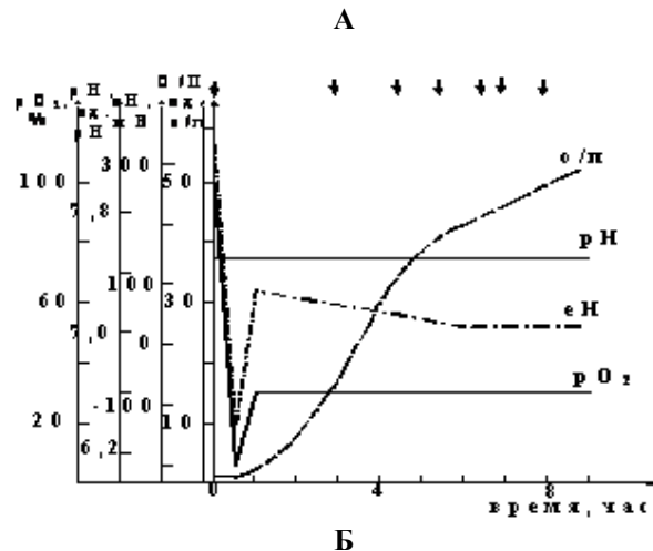
Рис. 2 - Динамика основных параметров культивирования листерий в режиме: А - инструкторном; Б - экспериментальном; pO_2 - парциальное давление растворенного кислорода; pH - концентрация водородных ионов; eH - окислительно - восстановительный потенциал; o/п - оптическая плотность; \tau - продолжительность культивирования; \downarrow - подача глюкозы
