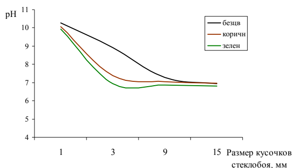
Рис. 1 - Зависимость pH водной вытяжки от размеров кусочков стеклобоя и сорта тарного стекла: 1-безцветное стекло, 2-коричневое стекло, 3-зеленое стекло
