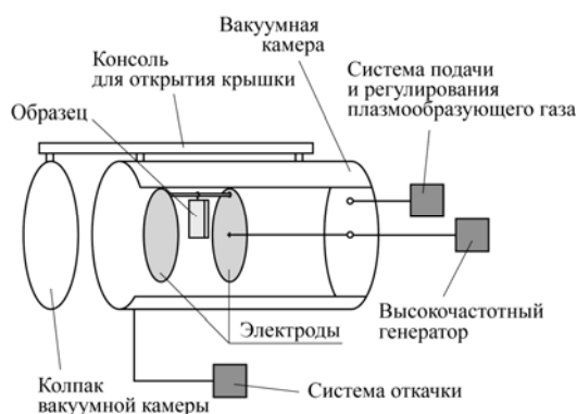
Рис. 1 – Схема высокочастотной емкостной плазменной установки барабанного типа
