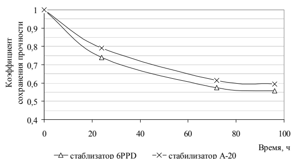
Рис. 1 – Изменение коэффициента сохранения прочности вулканизатов резиновых смесей
