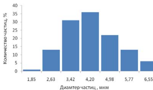
Рис. 2 - Гистограмма распределение композиционных частиц ибупрофен/ПЭГ 4000 по размерам
