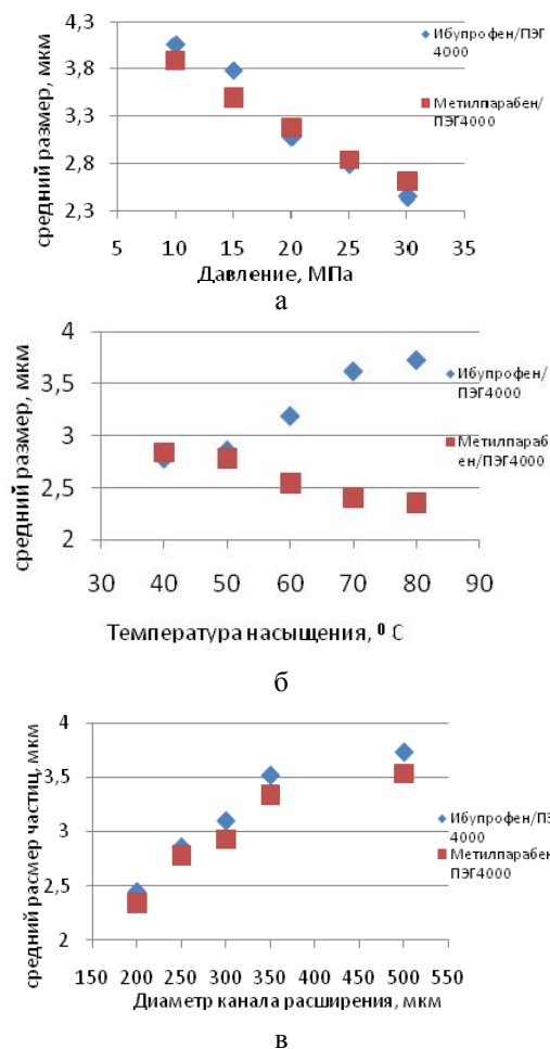
Рис. 3 - Зависимость среднего размера композиционных частиц от: а - давления насыщения; б - температуры насытителя; в - диаметра канала расширения
