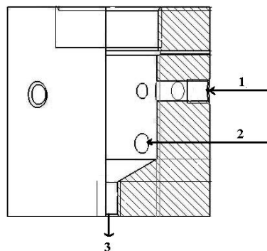
Рис. 1 - Ячейка для получения композиционных частиц: 1 – порт подачи CO 2 , 2 – термopapa, 3 – отверстие для отбора раствора
