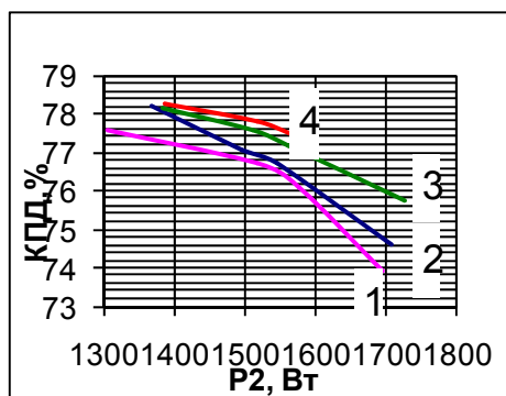
Рис. 3 – Зависимость КПД серийного (1) и опытных (2 - 4) асинхронных двигателей
