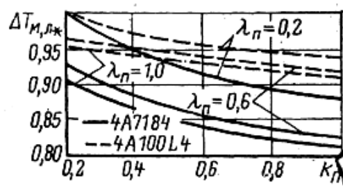
Рис. 2– Зависимость превышения температуры лобовой части обмотки статора со стороны привода двигателей серии 4А от коэффициента пропитки ( k_n ) и коэффициента теплопроводности пропиточного состава ( \lambda_n ), Вт/(м·К)
