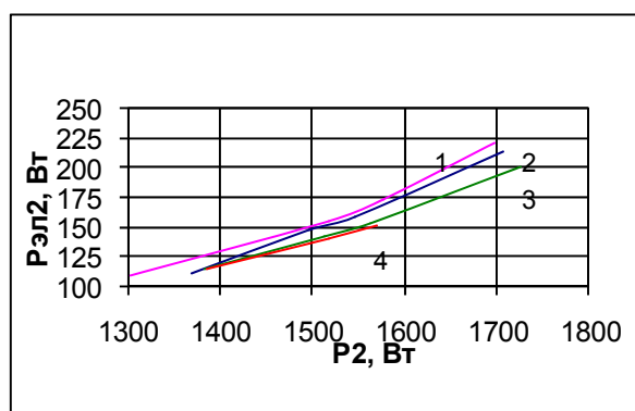
Рис. 4 – Зависимость электрических потерь в обмотке ротора серийного (1) и опытных (2 - 4) асинхронных двигателей
