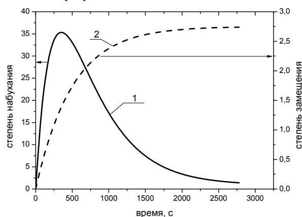
Рис. 1 - Зависимость степени набухания полимера (1) и степени замещения нитратов целлюлозы (2) от времени процесса. ( k = 100k_x )
