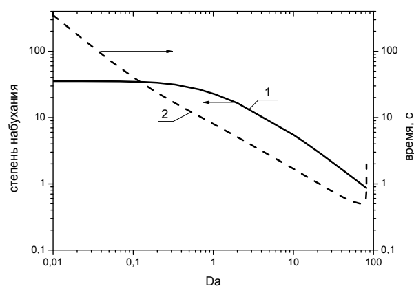
Рис. 4 - Зависимость максимальной степени набухания (1) и времени достижения максимального набухания (2) от критерия Дамкеллера-Дьяконова
