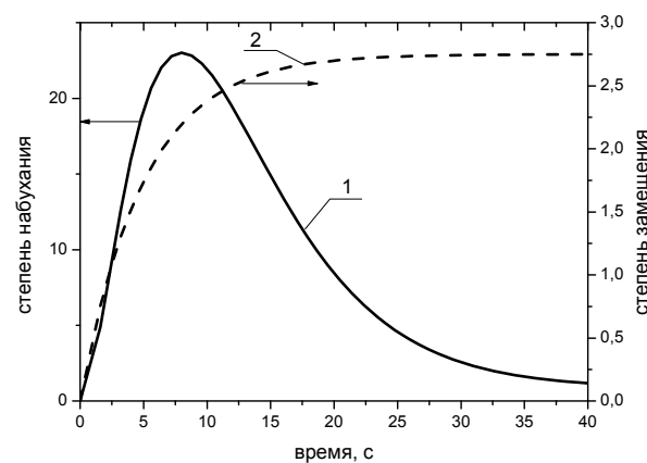
Рис. 2 - Зависимость степени набухания полимера (1) и степени замещения нитратов целлюлозы (2) от времени процесса. ( k = k_x )
