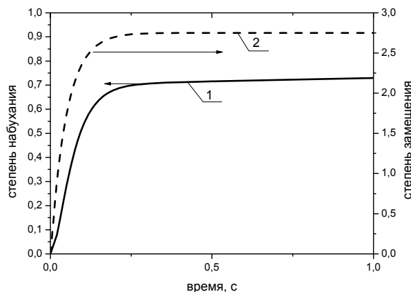
Рис. 3 - Зависимость степени набухания полимера (1) и степени замещения нитратов целлюлозы (2) от времени процесса. ( k=0,01k_x )
