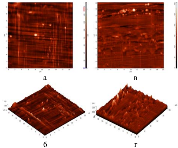
Рис. 2 – АСМ фотографии поверхности и 3D изображения исходных ПП мононитей марки PROLENE (США) (а, б) и марки USP 1 (Германия) (в, г)
