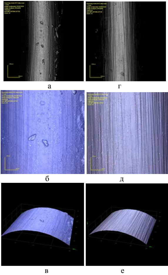
Рис. 1 – ЛСМ фотографии и 3D изображения исходных ПП мононитей марки PROLENE (США) (а, б, в) и ( г, д, е) марки USP 1 (Германия)
