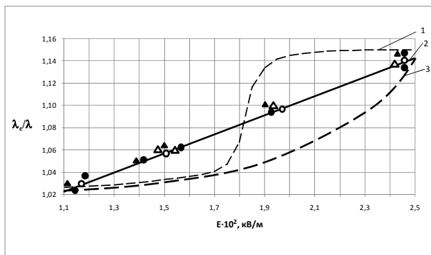
Рис. 1 – Зависимость относительного изменения коэффициента теплопроводности от напряженности электрического поля при частоте 5 \cdot 10^5 Гц: 1 – кривая, полученная на основе нейросетевой модели при \Delta \epsilon_s = 39 мВ; 2 – экспериментальная кривая [1], полученная после аппроксимации; 3 – кривая, полученная на основе математической модели [1]; ○, ●, ▲, △ - экспериментальные точки, соответствуют четырем различным значениям средних температур слоя жидкости, соответственно 17,0; 17,2; 17,4; 17,6°С
