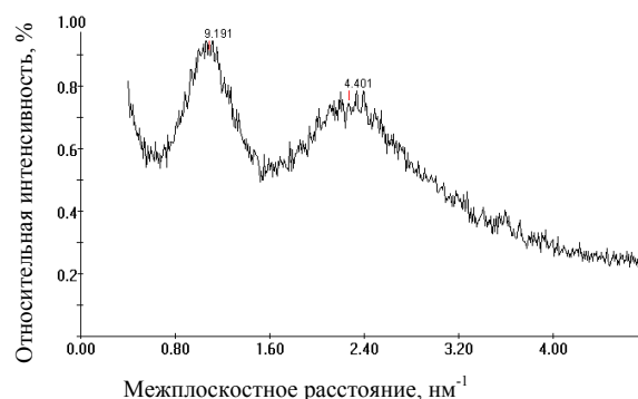
Рис. 1 – Дифрактограмма структуры пигментированного волосяного покрова шубной овчины после процесса осветления, контрольный образец
