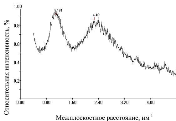
Рис. 2 – Дифрактограмма структуры пигментированного волосяного покрова шубной овчины после процесса осветления, опытный образец
