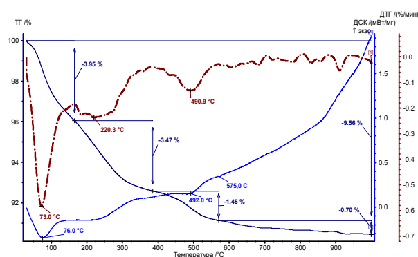
Рис. 1 - Термические кривые диатомита Ирбитского месторождения
