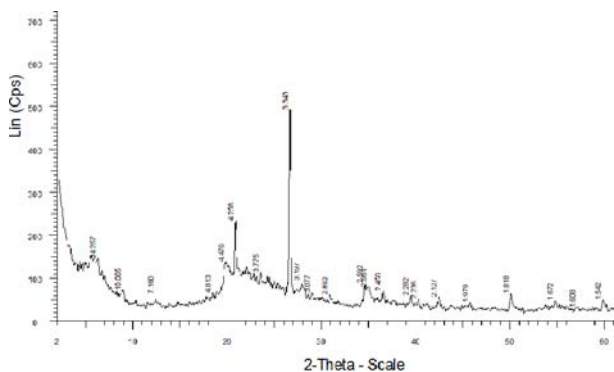
Рис. 2 - Рентгенограммы Ирбитского диатомита
