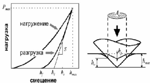
Рис. 2 - Общий вид кривой нагружения, и схема контакта с обозначениями величин, используемых в методике расчета модуля упругости и твердости
