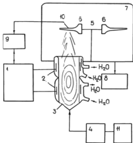
Рис. 1 - Установка ПУ-ВЧЕ для полировки и очистки: 1 – ВЧ-генератор, 2 – электроды, 3 – водоохлаждаемая РК, 4 – устройство очистки аргона, 5 – карусельное устройство, 6 – обрабатываемая деталь, 7 – вакуумная камера, 8 – система откачки, 9 – система контроля-управления, 10 – термопары, 11 – система газоснабжения
