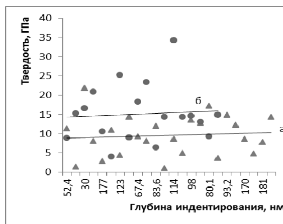
Рис. 5 - Изменение микротвердости поверхности сплава ВК8: а – образец до обработки, б – образец, обработанный в ВЧЕ плазме аргона, Q=2000 \text{ см}^3/\text{мин} , U=-20 \text{ В}
