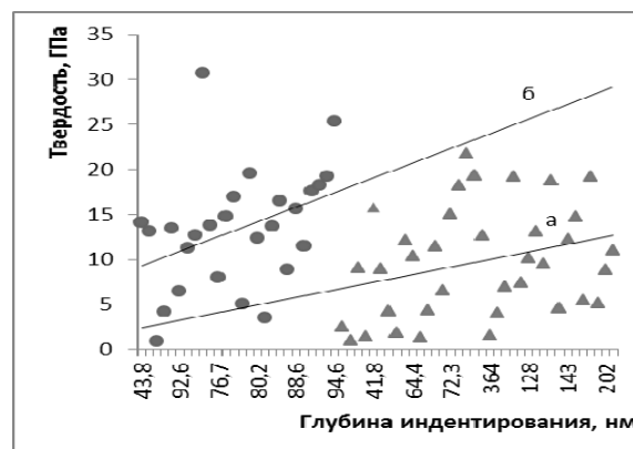
Рис. 6 - Изменение микротвердости поверхности сплава ВК8: а – образец до обработки, б – образец, обработанный по режиму Ar+C_3H_8 , Q_1=2000 \text{ см}^3/\text{мин} , Q_2=1400 \text{ см}^3/\text{мин} , U=-20 \text{ В}
