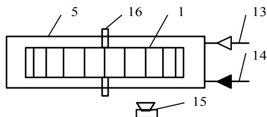
Рис. 2 – Схема экспериментальной установки (вид сверху): 1 – ротор; 5 – корпус; 13 – устройство для введения газового индикатора; 14 – устройство для введения жидкого индикатора; 15 – видеокамера; 16 – вал
