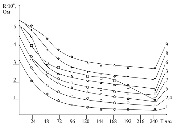
Рис. 1 - Изменение величины поляризационного сопротивления покрытий по времени в 3% растворе NaCl: 1,2,3 – покрытие №1 (толщина 0,1;0,5;1,0мм); 4,5,6 покрытие №2 (толщина 0,1;0,5;1,0мм); 7,8,9 покрытие №3 (толщина 0,5;1,0;2,0мм)
