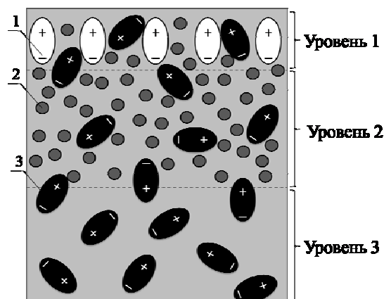
Рис. 2 - Модель распределения гомо- и гетерозарядов в полилактиде: 1 – диполи, образованные в результате окисления поверхности; 2 – инжектированные носители заряда; 3 – диполи в объеме полимера
