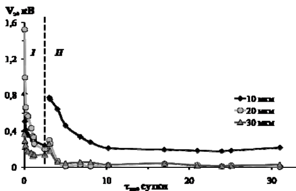
Рис. 1 - Изменение потенциала поверхности двухслойных коронозлектретов ПЛА – ПЭТФ при хранении до (область I) и после удаления (область II) верхнего слоя полилактида
