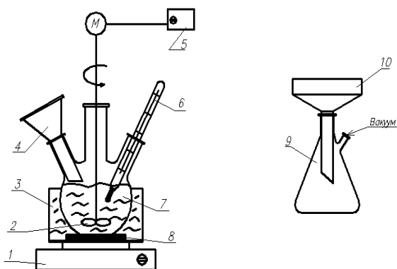
Рис. 1 – Схема лабораторной установки (реактор 3 л): 1 – электроплитка; 2 – мешалка; 3 – водяная баня; 4 – воронка; 5 – ЛАТР; 6 – термометр; 7 – трёхгорлая колба; 8 – прокладка; 9 – колба Бунзена; 10 – вакуум-воронка Бюхнера
