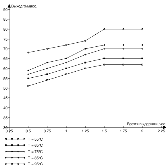
Рис. 4 - Зависимость выхода аспарагината марганца от температуры и времени выдержки при навеске углекислого марганца 0,200 кг
