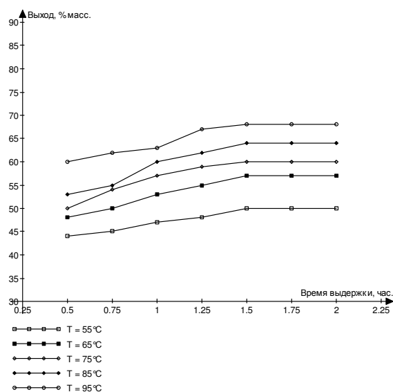
Рис. 2 – Зависимость выхода аспарагината марганца от температуры и времени выдержки при навеске углекислого марганца 0,184 кг
