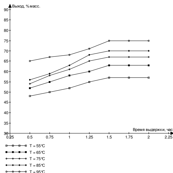
Рис. 3 – Зависимость выхода аспарагината марганца от температуры и времени выдержки при навеске углекислого марганца 0,190 кг
