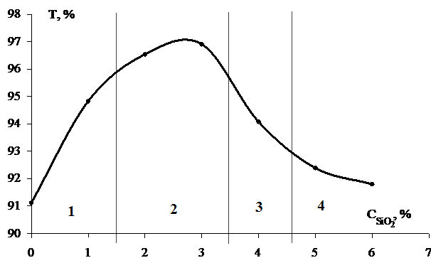
Рис. 2 - Зависимость светопропускания ( \lambda=540\text{нм} ) стеклянных образцов с покрытием от концентрации диоксида кремния
