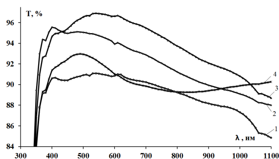
Рис. 1 – Спектры пропускания стеклянных образцов с покрытием, полученным из золя диоксида кремния с концентрацией: 1 – стекло без покрытия; 2 – 1%; 3 – 3%; 4 – 5%
