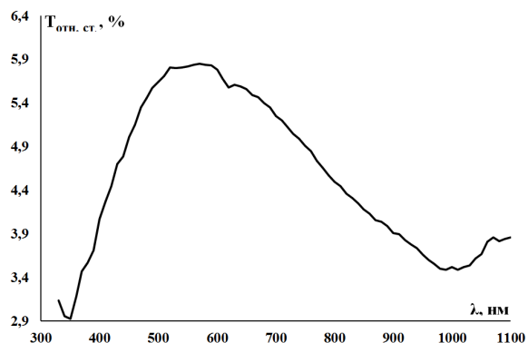
Рис. 4 – Изменение оптического пропускания стекла с просветляющим покрытием на основе сферических частиц SiO_2 относительно стекла без покрытия ( \Delta T = T_{\text{стекло с покрытием}} - T_{\text{стекло}} ) при угле падения излучения на образец, близком к нормальному
