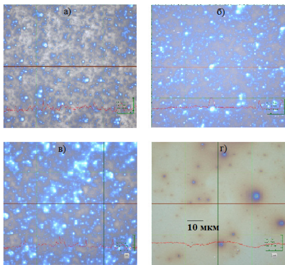
Рис. 3 - Микрофотографии покрытий из золь-гелей диоксида кремния с разной концентрацией: а) 1%, б) 3%, в) 5%, г) 10%
