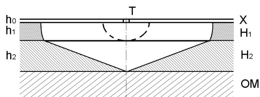
Рис. 1 - Коррозионные очаги в слоях биникель хромовом покрытии с микротрещиноватым хромовым слоем ( X_{\text{мтр}} )
