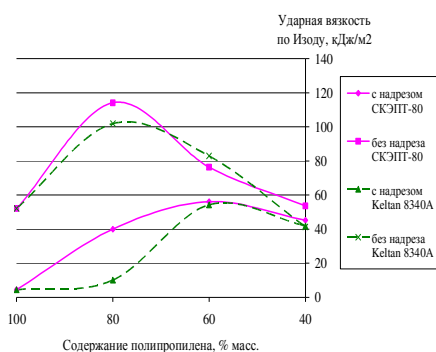
Рис. 2 – Ударная вязкость термоэластопластов на основе ПП 1500J при комнатной температуре
