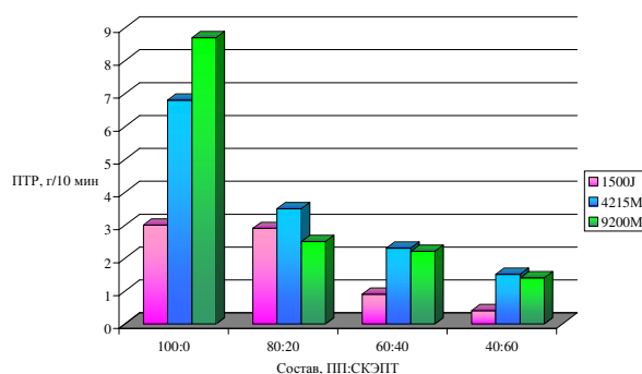
Рис. 1 – Изменение показателя текучести расплава термоэластопластов в зависимости от состава (на основе СКЭПТ-80)
