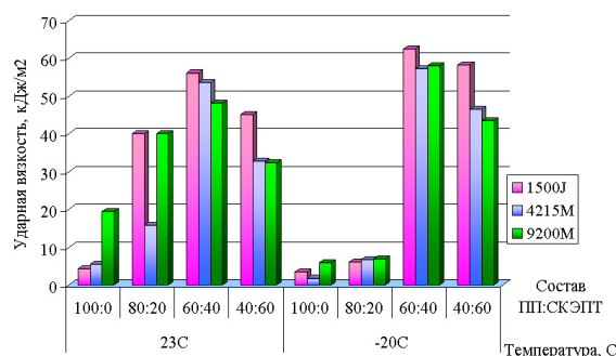
Рис. 3 – Ударная вязкость термоэластопластов на основе СКЭПТ-80 (для образцов с надрезом)
