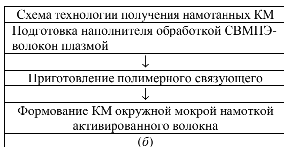
Рис. 2 - Схемы технологий получения КМ с применением обработки волокнистых наполнителей ННТ плазмой: а – слоистых и б – намотанных нетканых композитов
