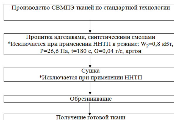
Рис. 3 – Вариант технологической схемы модификации технических тканей с повышенной адгезией с помощью плазменной обработки
