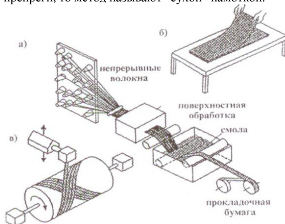
Рис. 1 - Изготовление слоистых намотанных КМ с полимерной матрицей: а – общая схема изготовления КМ; б – схема изготовления многослойного листового КМ; в – схема изготовления многослойного намотанного КМ.
