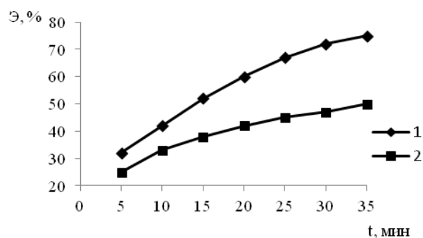
Рис. 4 - Зависимость эффективности очистки модельных раствора МГ от интенсивности перемешивания: 1 – масса добавки ИКК 2,5 г на 100 мл раствора, 2 – масса добавки ИКК 1,0 г на 100 мл раствора
