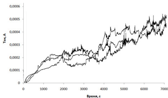
Рис. 1 - Потенциостатические поляризационные кривые стали марки 12X18H10T в растворе 0,1 М NaCl
