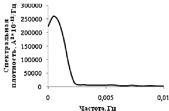
Рис. 3 - График спектральной плотности флуктуаций тока для области существования метастабильных питтингов
