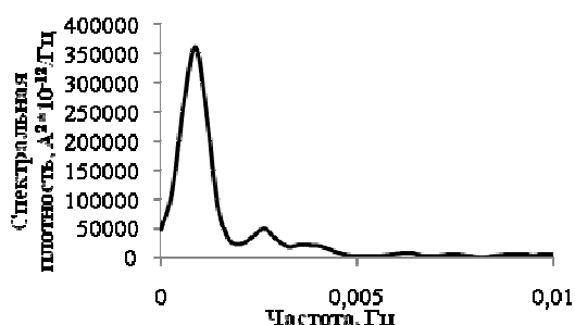
Рис. 4 - График спектральной плотности для области существования метастабильных и стабильных питтингов
