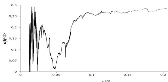
Рис. 2 - Временная зависимость отношения стандартного отклонения силы тока \sigma(I) к его среднему значению \langle I \rangle стали марки 12X18H10T в растворе 0,1 М NaCl
