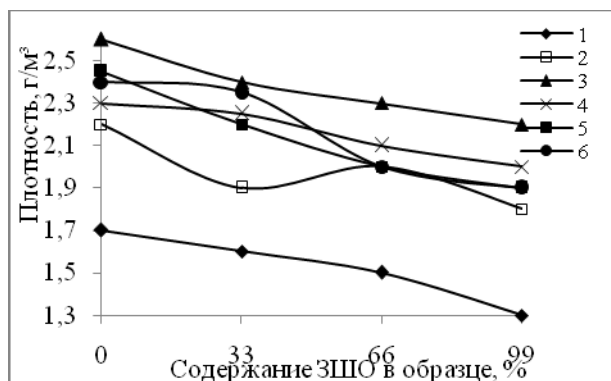
Рис. 2 - Зависимость плотности образцов от процентного содержания ЗШО в образцах: 1 - без пропитки серой; 2 - пропитанных чистой серой; 3 - образцы пропитанные в серном расплаве с содержанием 1%Na 2 SiO 3 ; 4 - то же самое, 3%Na 2 SiO 3 ; 5 - образцы, пропитанные в серном расплаве, содержащем 1%AlCl 3 ; 6 - то же самое, 5%AlCl 3
