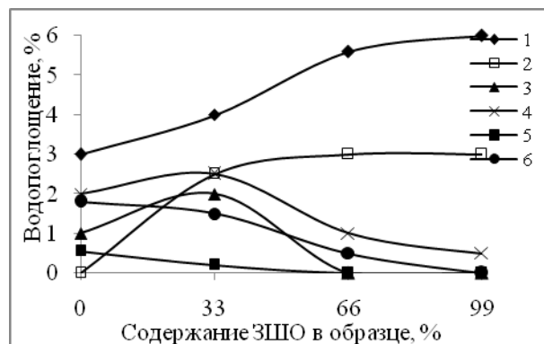
Рис. 2 - Зависимость водопоглощения образцов от процентного содержания ЗШО в образцах: 1 – без пропитки серой; 2 – пропитанных чистой серой; 3 – образцы пропитанные в серном расплаве с содержанием 1% \text{Na}_2\text{SiO}_3 ; 4 – то же самое, 3% \text{Na}_2\text{SiO}_3 ; 5 – образцы пропитанные в серном расплаве, содержащем 1% \text{AlCl}_3 ; 6 – то же самое, 5% \text{AlCl}_3
