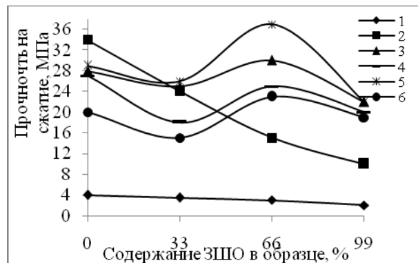
Рис. 1 - Зависимость прочности образцов от содержания ЗШО в образцах: 1 – без пропитки серой; 2 – пропитанных чистой серой; 3 – образцы пропитанные в серном расплаве с содержанием 1% \text{Na}_2\text{SiO}_3 ; 4 – то же самое, 3% \text{Na}_2\text{SiO}_3 ; 5 – образцы пропитанные в серном расплаве, содержащем 1% \text{AlCl}_3 ; 6 – то же самое, 5% \text{AlCl}_3
