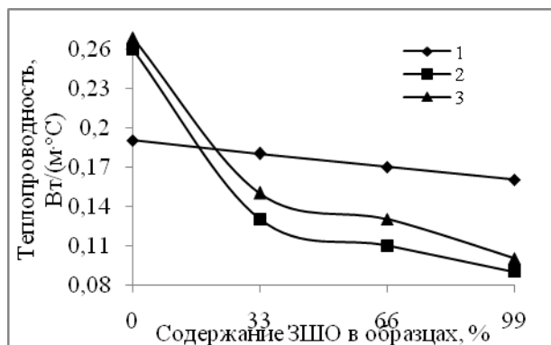
Рис. 4 - Зависимость теплопроводности образцов от процентного содержания ЗШО: 1 - образцы без пропитки серой; 2 - образцы, пропитанные в серном расплаве сNa 2 SiO 3 ; 3 - образцы, пропитанные в серном расплавеAlCl 3
