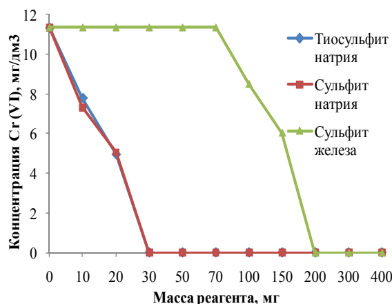
Рис. 4 – Восстановление хрома (VI) с помощью железной стружки в смеси с традиционными реагентами
