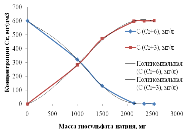
Рис. 1 – Восстановление Cr 6+ до Cr 3+ с использованием тиосульфата натрия
