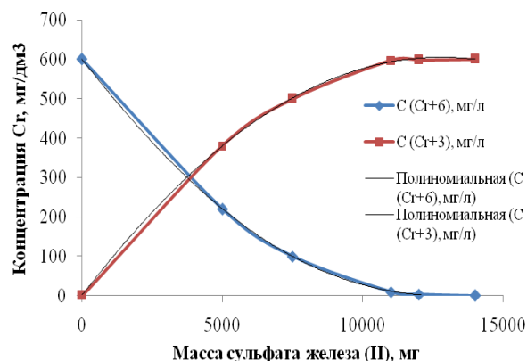
Рис. 2 – Восстановление Cr 6+ до Cr 3+ с использованием сульфата железа (II)
