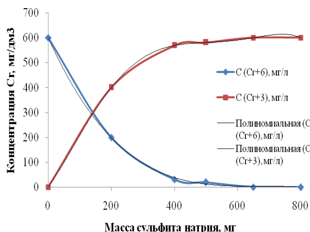
Рис. 3 – Восстановление \text{Cr}^{6+} до \text{Cr}^{3+} с использованием сульфита натрия
