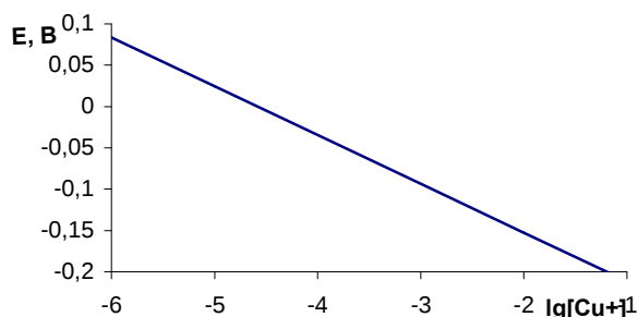
Рис. 2 - Расчетная зависимость потенциала платинового электрода от концентрации ионов меди (1)
