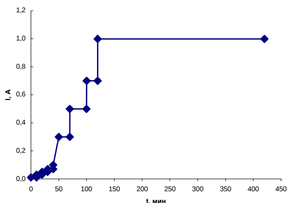
Рис. 3 - Зависимость силы тока от времени затяжки образца
