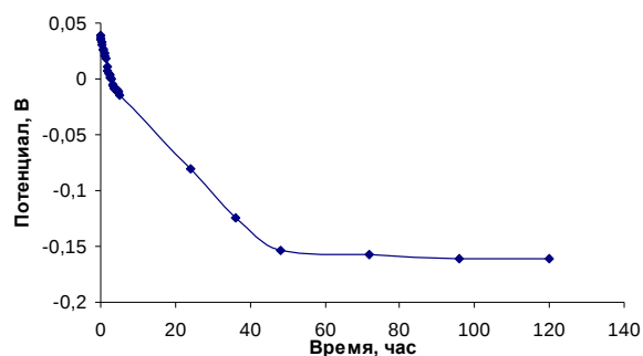
Рис. 1 - Изменение потенциала платинового электрода в растворе сорбции
