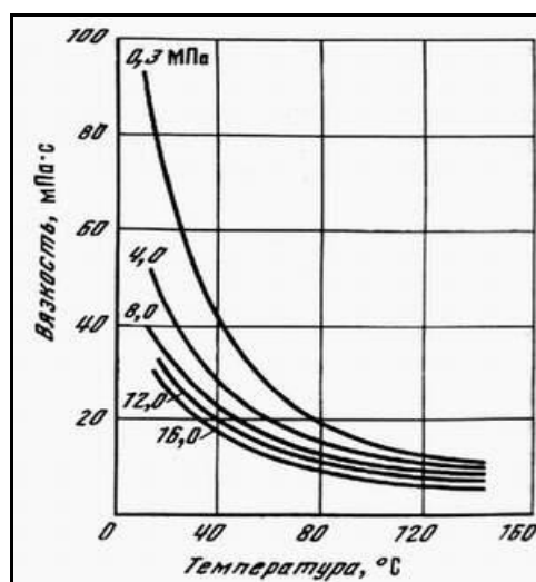
Рис. 1 - Зависимость вязкости нефти от давления и температуры [3]
