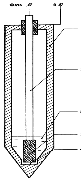
Рис. 2 - Скважинный ионный нагреватель: 1 - металлический корпус; 2 - центральный электрод; 3 - изолятор; 4 - упор; 5 - электролит
