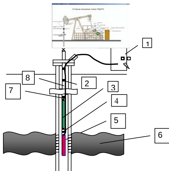
Рис. 3 - Расположение ионного нагревателя в скважине: 1- блок управления, 2 - клипсы крепления кабеля, 3 - насос ШГН, 4 – фильтр, 5 – ионный нагреватель, 6 - нефтяной пласт, 7 - кабель КРБК, 8 – насосно-компрессорная труба
