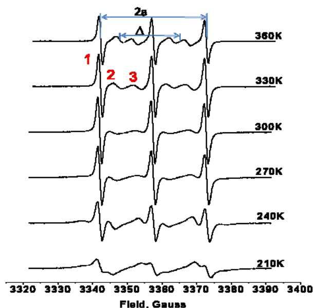
Рис. 2 – Температурная зависимость спектров бирадикала ТЕМРМ
