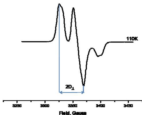
Рис. 4 - Спектр застеклованного раствора для бирадикала ТЕМРМ
