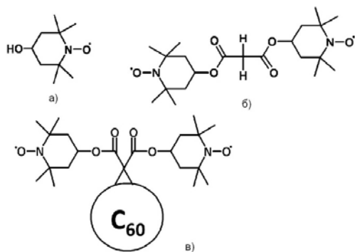
Рис. 1 - Структурные формулы: а) ТЕМРО; б) ТЕМРМ; в) ТЕМРФ
