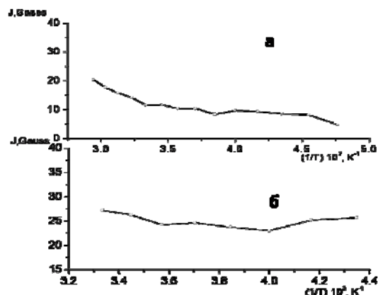
Рис. 3 - Температурная зависимость измеряемого значения обменного интеграла J для а) ТЕМРМ, б) ТЕМРФ
