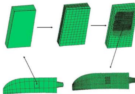
Рис. 2 – Конечно-элементная модель лопасти
