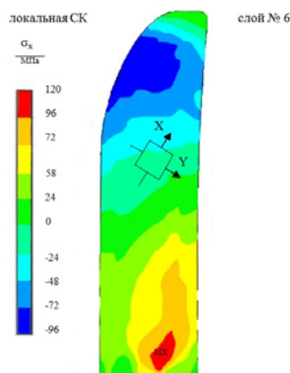
Рис. 3 — Пример расчета НДС лопасти
