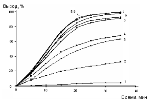
Рис. 1 – Конверсионные кривые синтеза стеарата кальция в среде вода-ацетон (50 °C). Содержание ацетона в дисперсионной среде (% масс.) 1 – 100; 2 – 95; 3 – 80; 6 – 60; 7 – 50; 8 – 30; 9 – 20; 5 – 10; 4 – 5.
