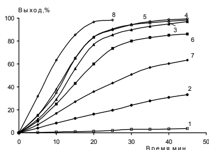
Рис. 2 – Конверсионные зависимости синтеза стеарата кальция в среде вода:изопропиловый спирт (50°C). Содержание изопропилового спирта в дисперсионной среде (% масс.): 1 - 100; 2 - 95; 3 - 50; 4 - 30; 5 - 20; 6 - 10; 7 - 5; 8 - 20 (70 °C).
